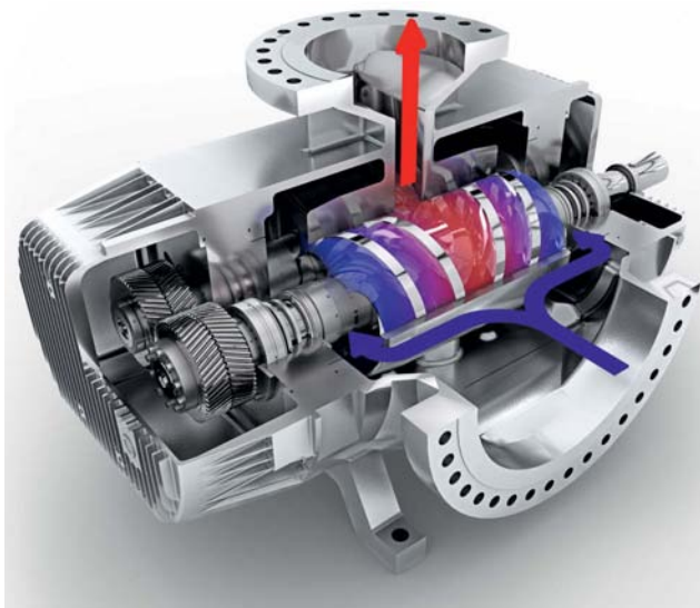
Leistritz L4NC pump
